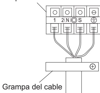
Bloque de terminal de la unidad interior
