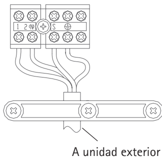
Bornera de la unidad interior
