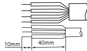
Bornera de la unidad exterior
