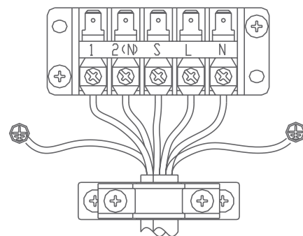
Bornera de la unidad exterior
